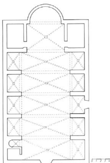
Plànol de l'Església de la Concepció de Caimari.
