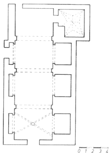
Plànol de l'Església de Sta. Tecla de Biniameu.
